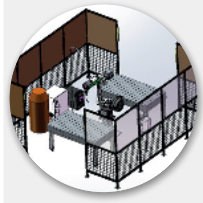
Роботизированная сварочная ячейка с двумя стационарными сварочными столами
