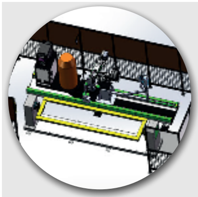
Роботизированная сварочная ячейка с одноосевым поворотным позиционером
