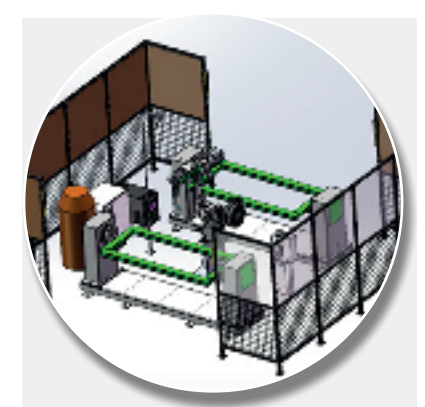
Роботизированная сварочная ячейка с двумя одноосевыми поворотными позиционерами
